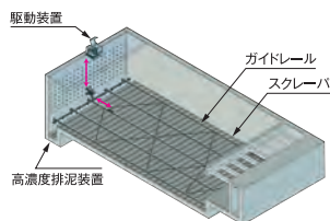
レシプロ式スラッジ掻き機+高濃度排泥装置
